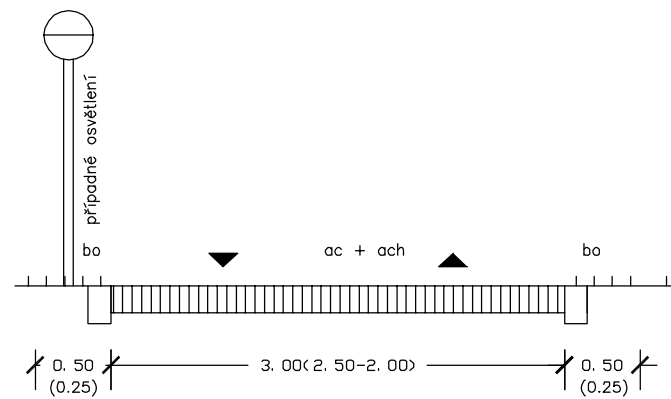
OBRÁZEK 68 – SPOLEČNÉ OBOUSMĚRNÉ STEZKY PRO CYKLISTY A CHODCE (při intenzitě menší 150 cyklistů/h a 180 chodců/h v obou směrech při menších intenzitách možno šířku zmenšit na 2,50 až na 2,00 m)
