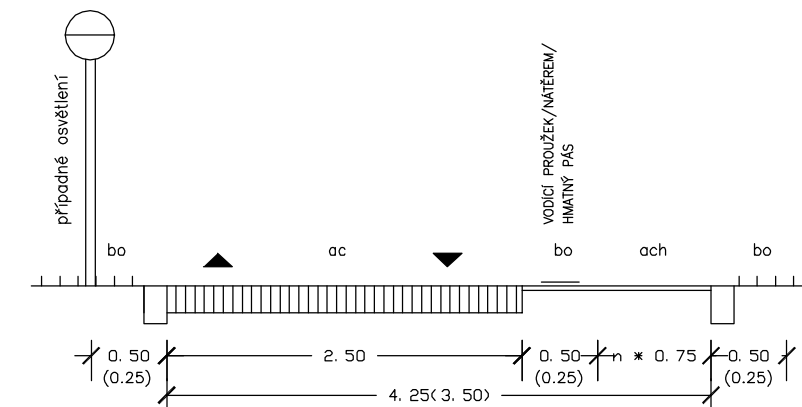
OBRÁZEK 67 – SOMOSTATNÁ STEZKA PRO CYKLISTY A CHODCE (obousměrný pás pro cyklisty)
