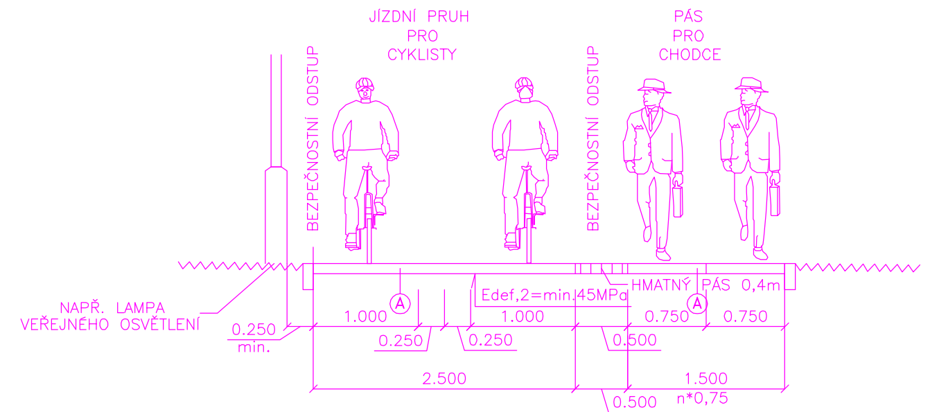
SCHEMA DLE ČSN 73 6110
